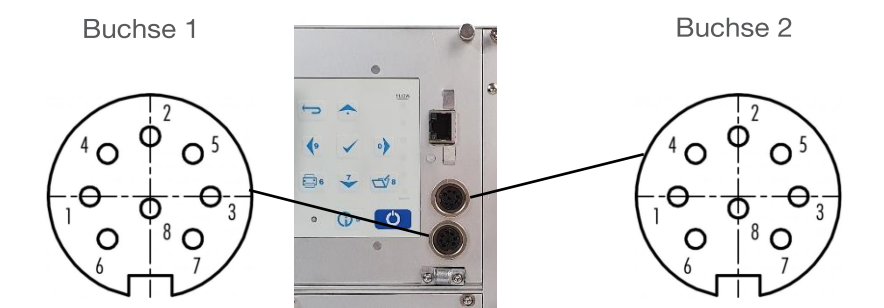
Anschlussbelegung Buchse 1
